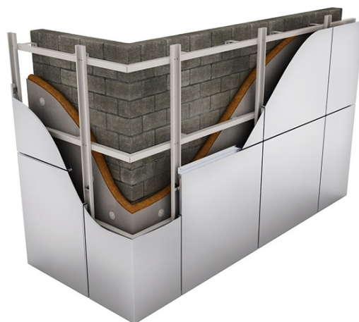
Горизонтально-вертикальная система крепления (кассетный способ)
