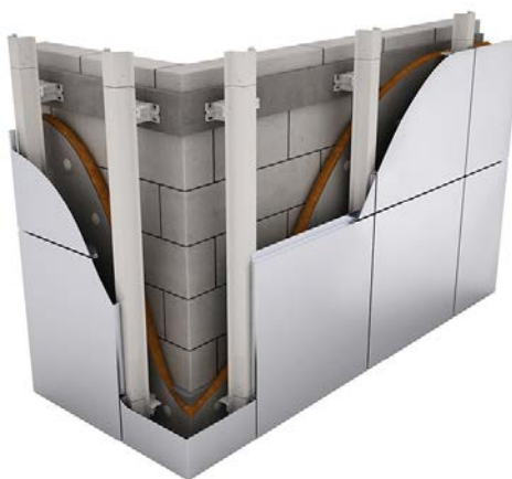
Система крепления в межэтажные перекрытия на основе кронштейна КНс-27 (кассетный способ)
