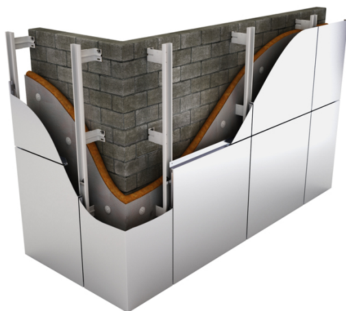
Вертикальная система крепления на основе С-образного профиля (кассетный способ)
