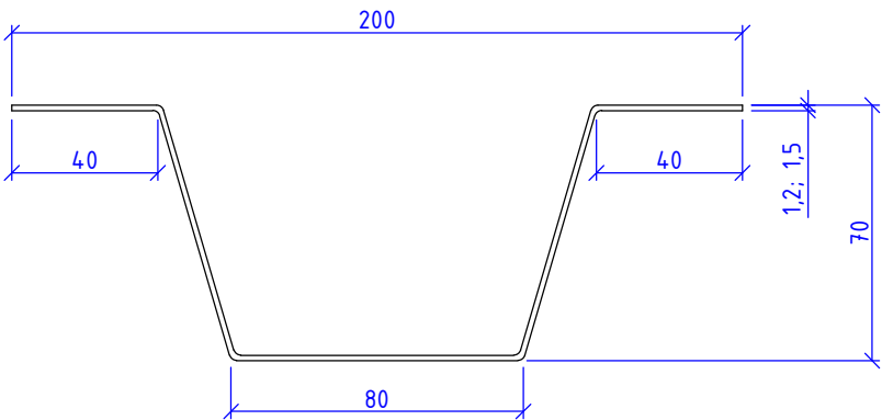
Вид спереди
