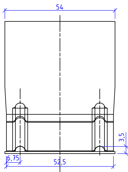
Вид спереди
