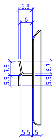
Вид сбоку
