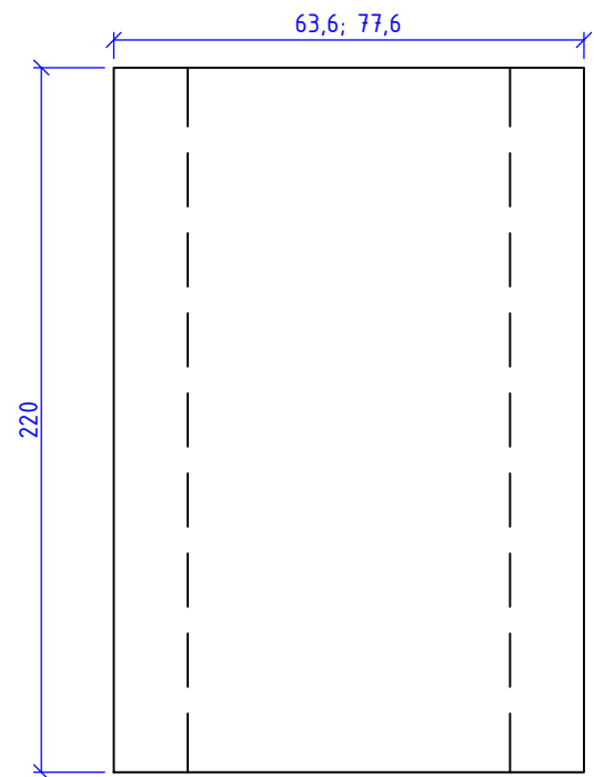
Вид спереди
