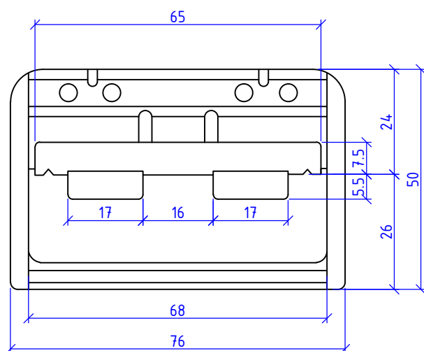
Вид спереди
