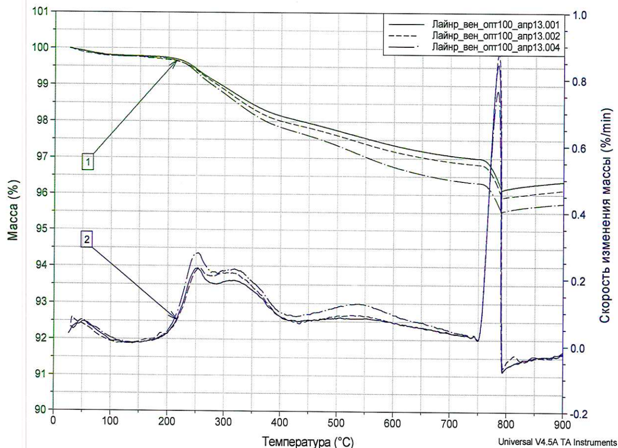
Рис.1. Термогравиметрические кривые образцов плиты минераловатной теплоизоляционной марки ЛАЙНРОК ВЕНТИ ОПТИМАЛ толщиной 100 мм, отобранной с навесной фасадной системы «АЛЪТ-ФАСАД-04»
