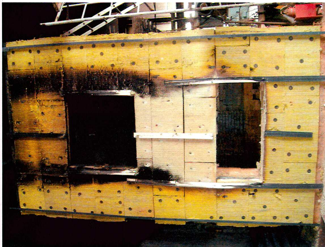
Фото №4 (вид образца после вскрытия конструкции)
