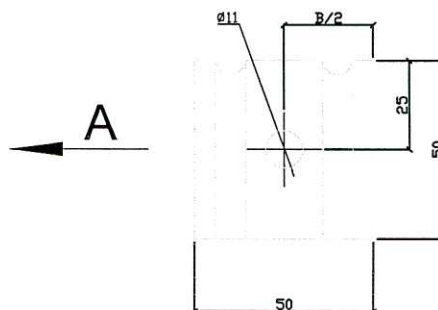
Вид А
