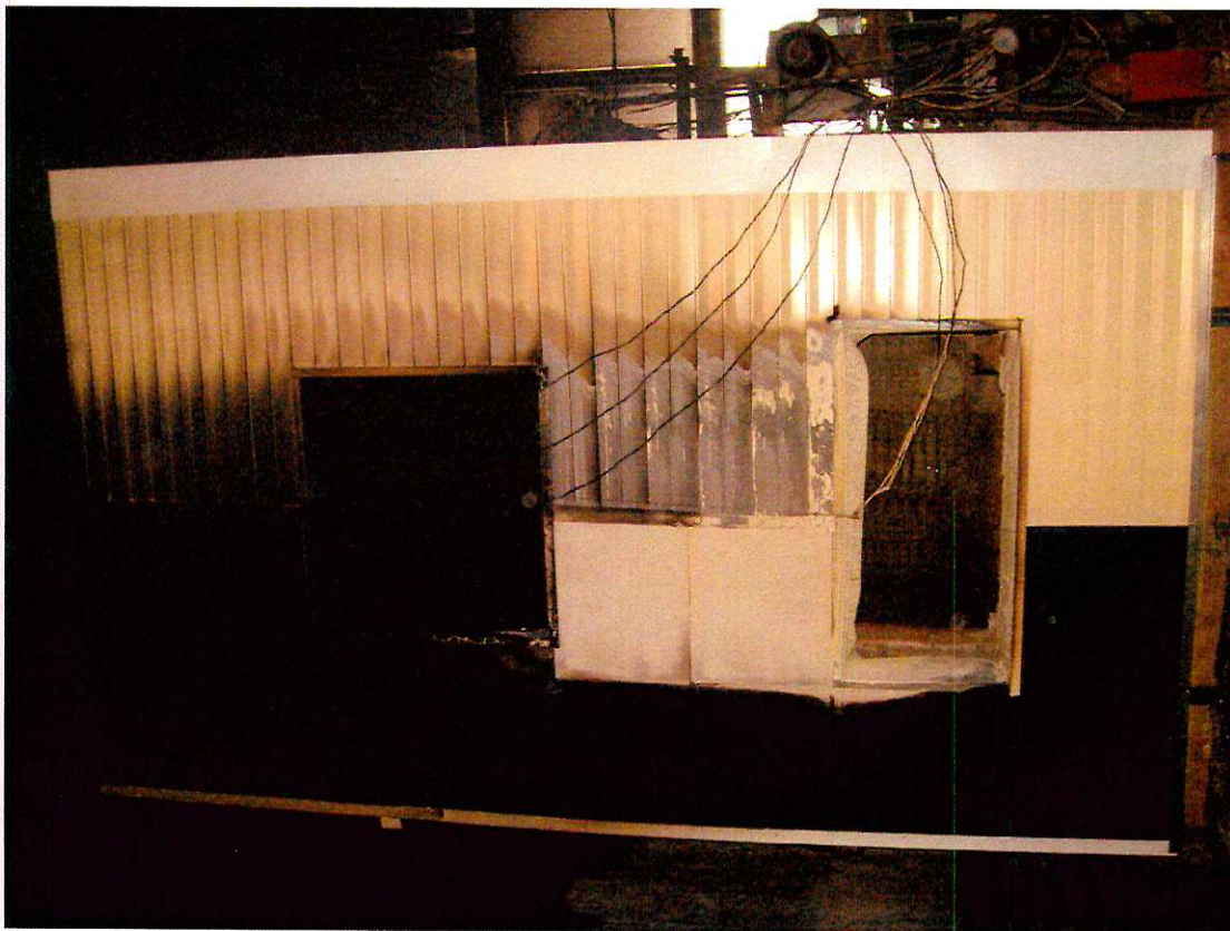
Фото №3 (вид образца после окончания испытания)
