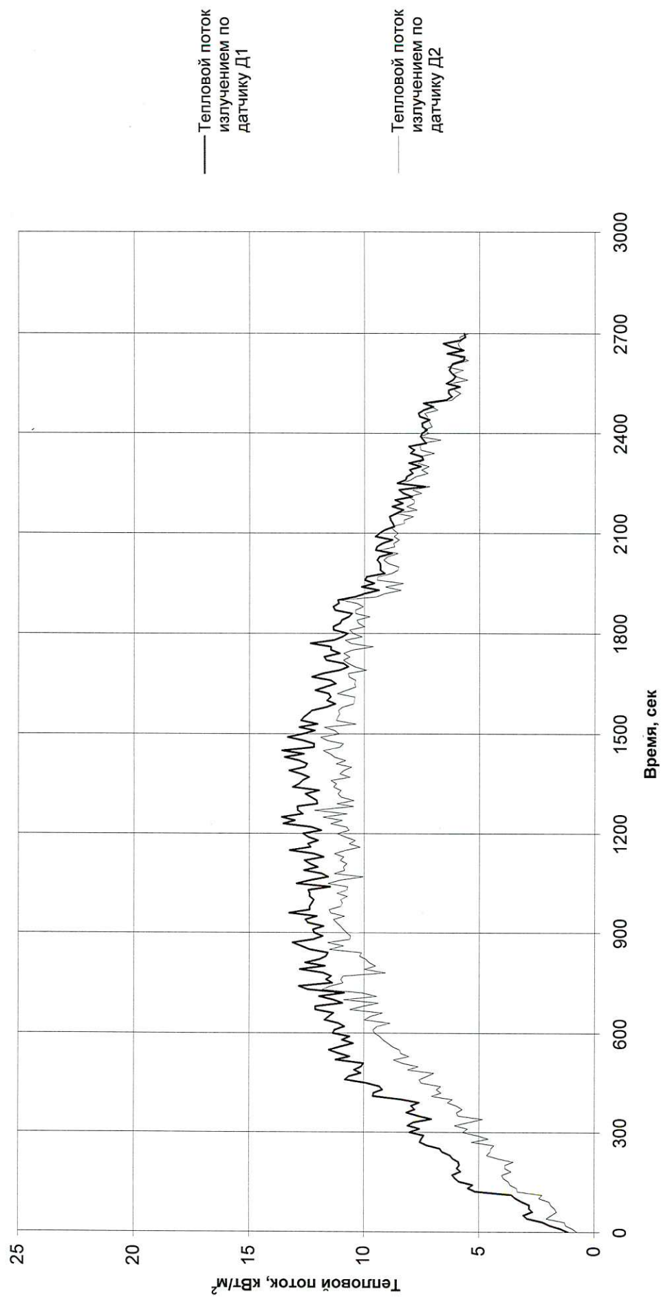
Рис. 36. Изменение во времени теплового потока при испытании образца
