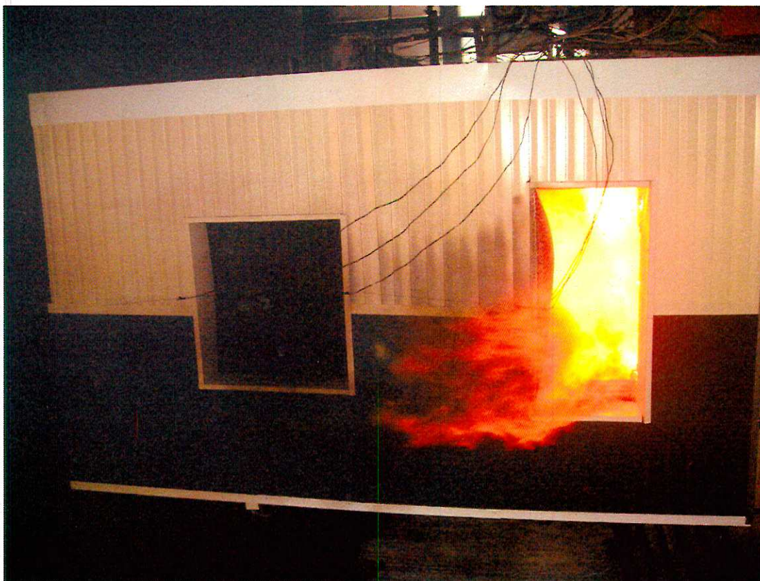
Фото №2 (8 мин испытания)
