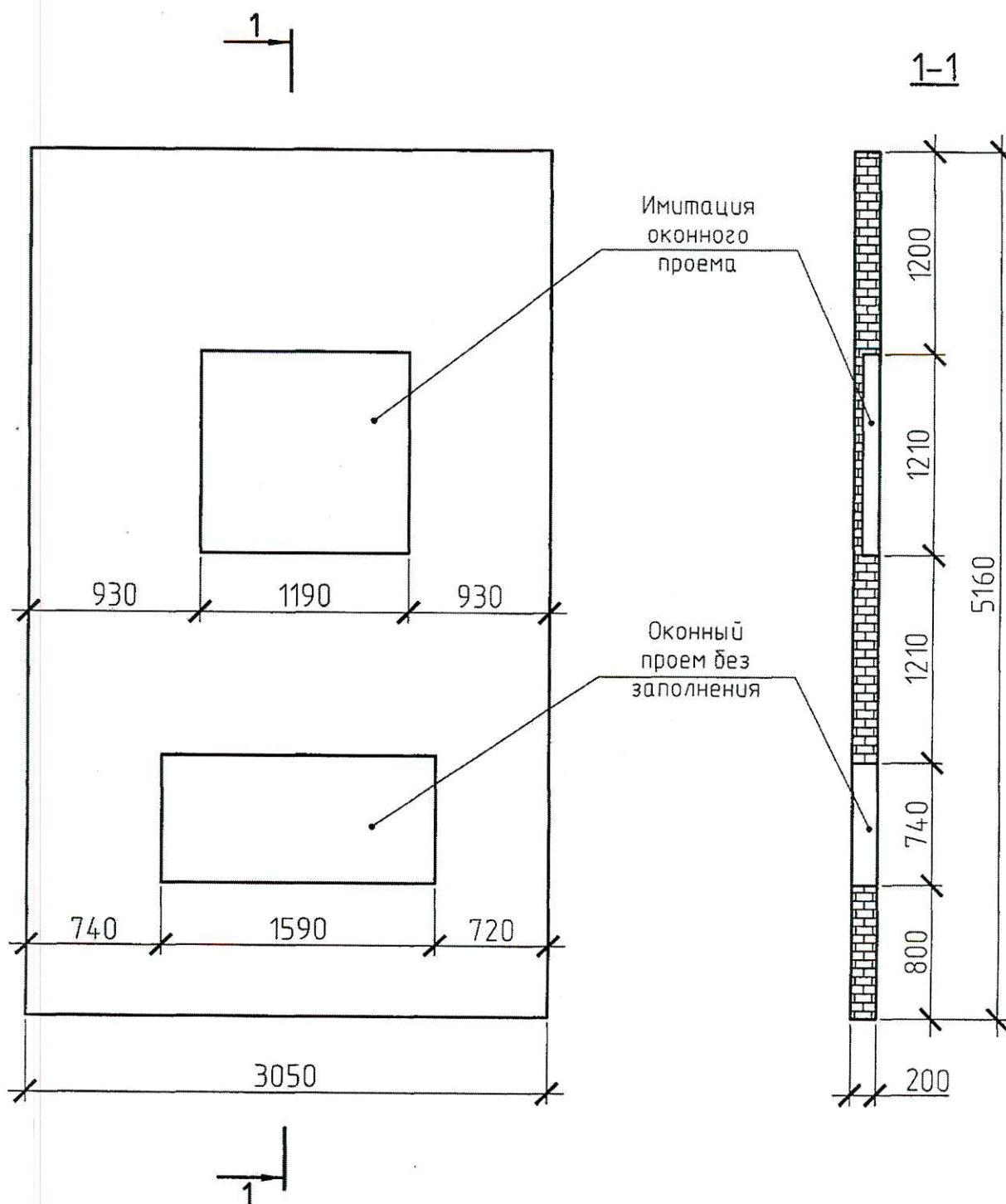
Рис. 1а. Схема фрагмента стены испытательного стенда
